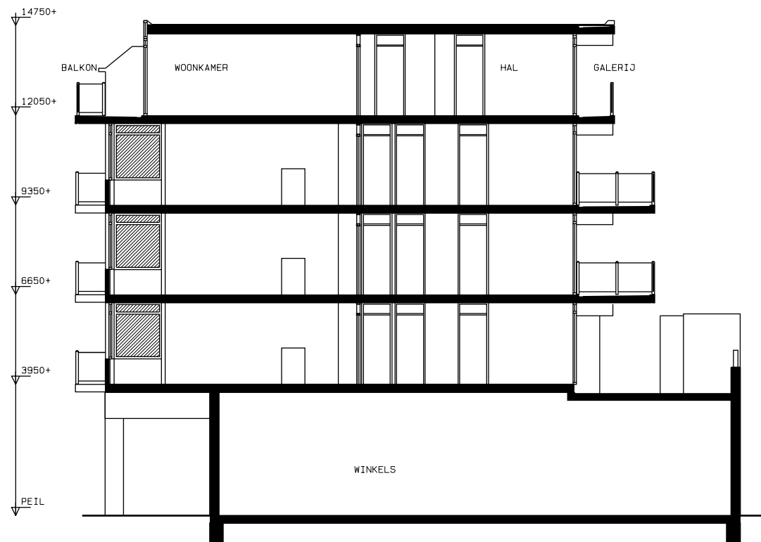
DOORSNEDE
