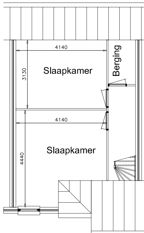
1e verdieping
