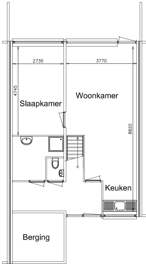
Begane grond
