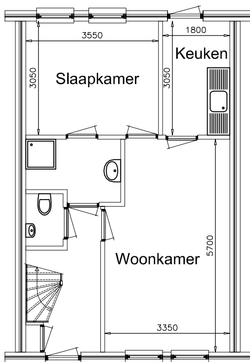
Begane grond
