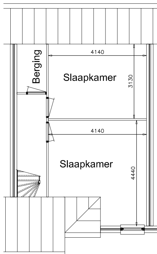
1e verdieping
