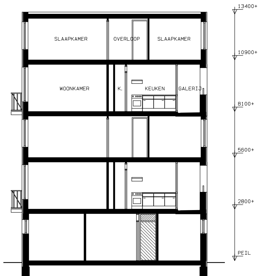
DOORSNEDE
