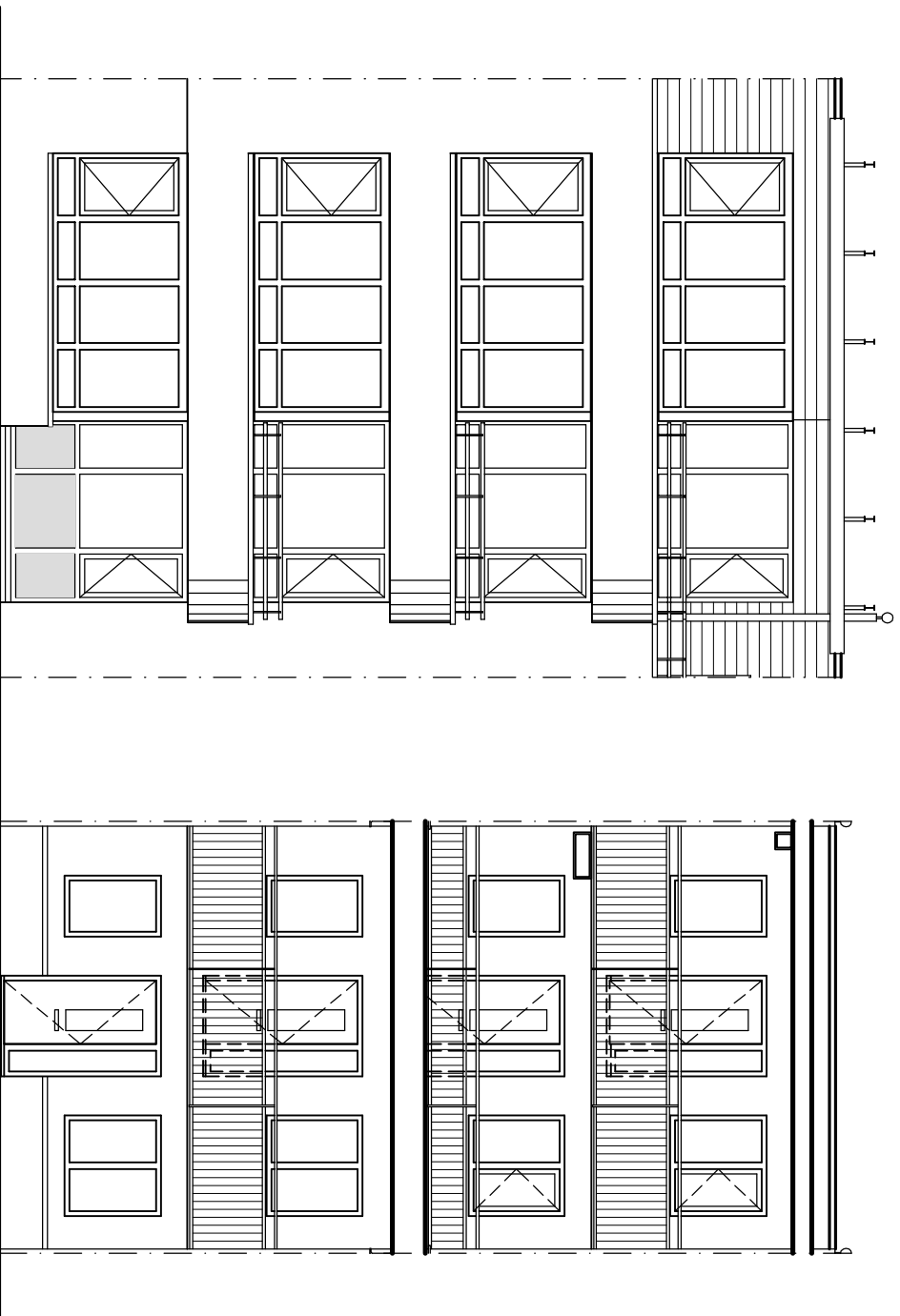
Voorgevel
