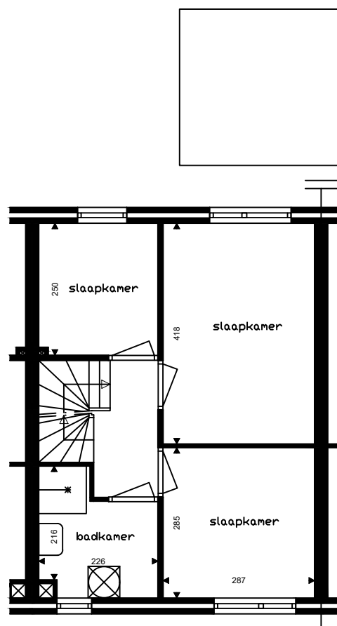
1e verdieping
