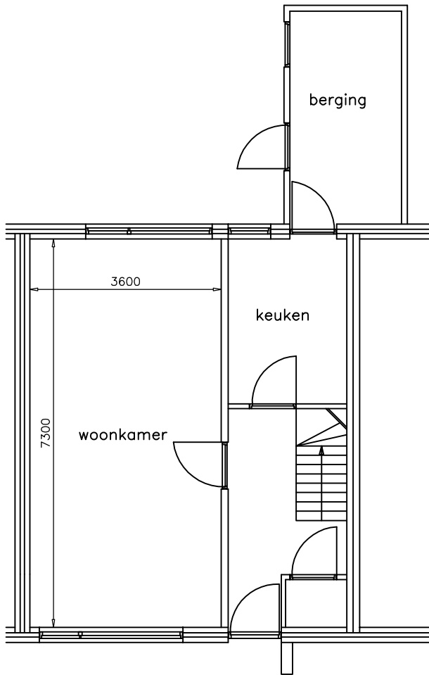
begane grond
