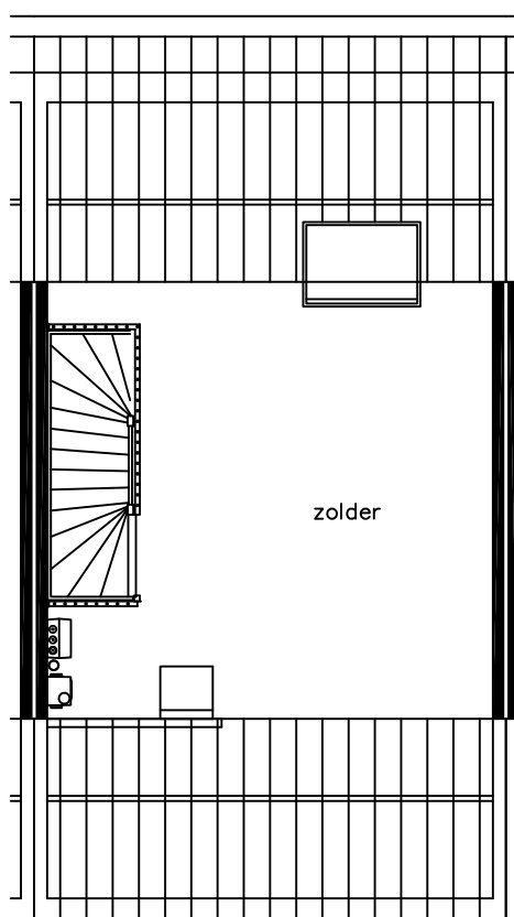
2e verdieping
