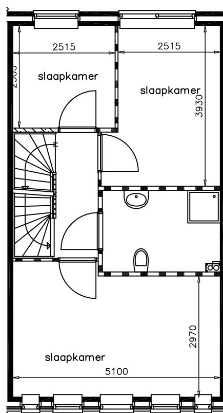
1e verdieping
