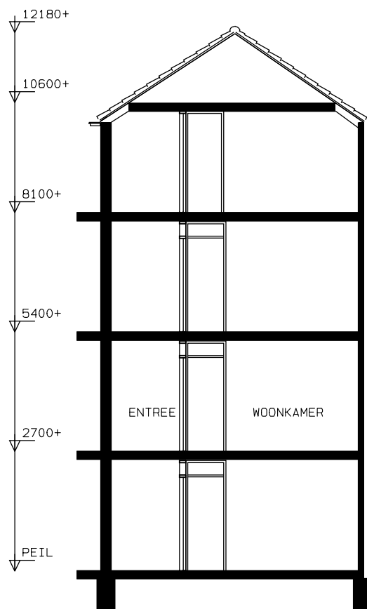
DOORSNEDE
