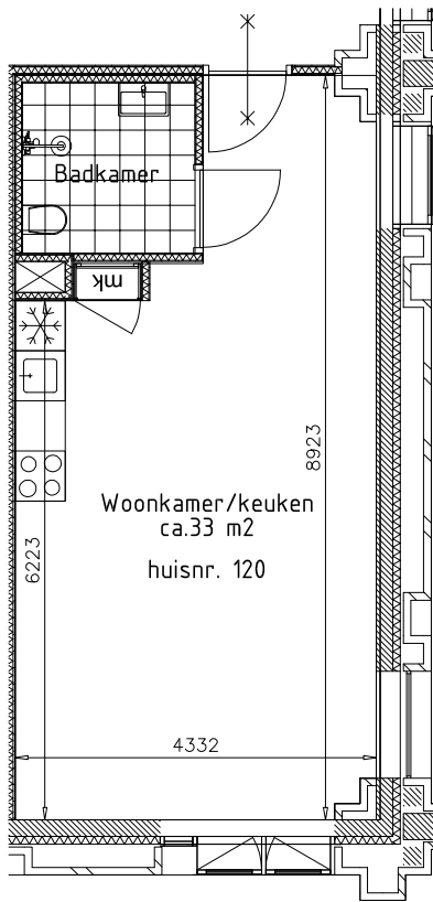
1e verdieping
