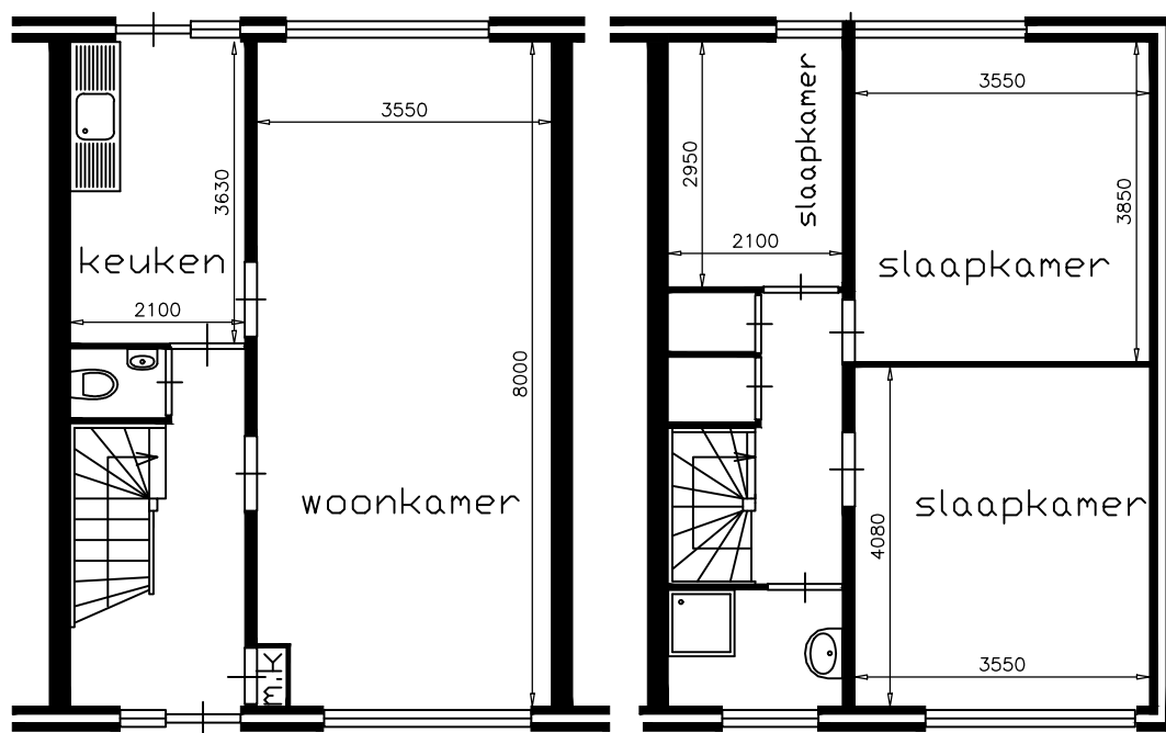
Begane grond
