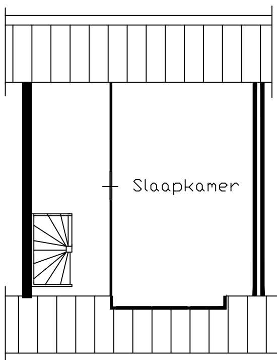
2e verdieping
