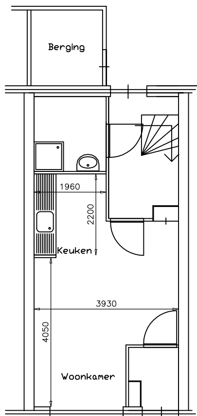
Begane grond
