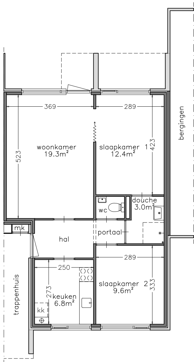
begane grond woningtype A
