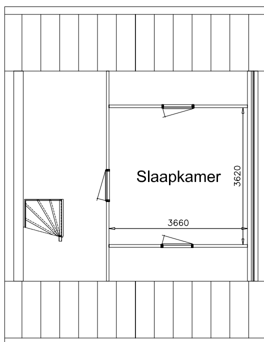
2e verdieping
