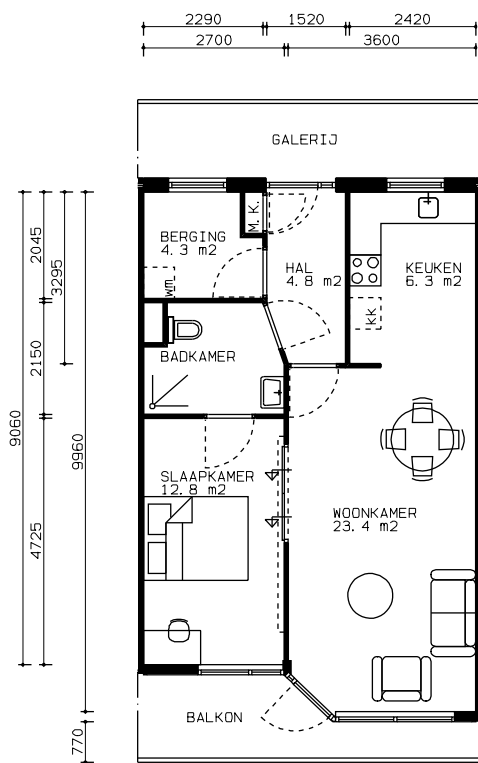
1e VERDIEPING
