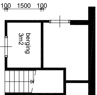
Begane grond
