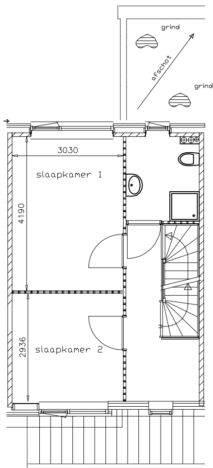
1e verdieping
