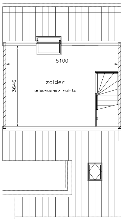
2e verdieping
