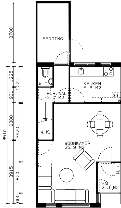
BEGANE GROND
