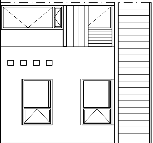
Voorgevel
