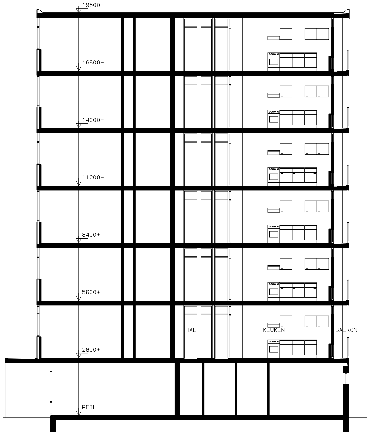
DOORSNEDE
