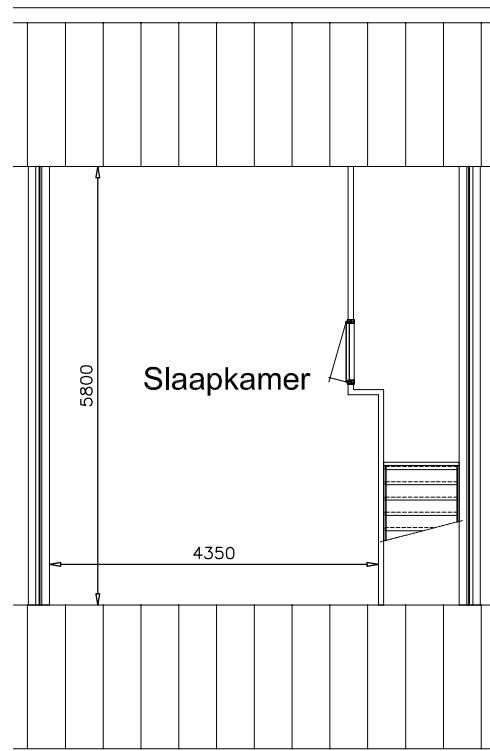
1e verdieping
