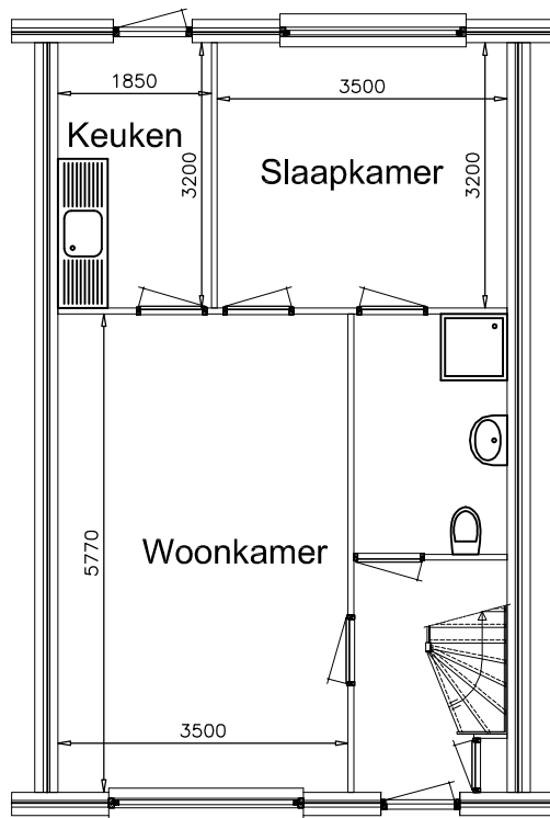
Beganegrond
