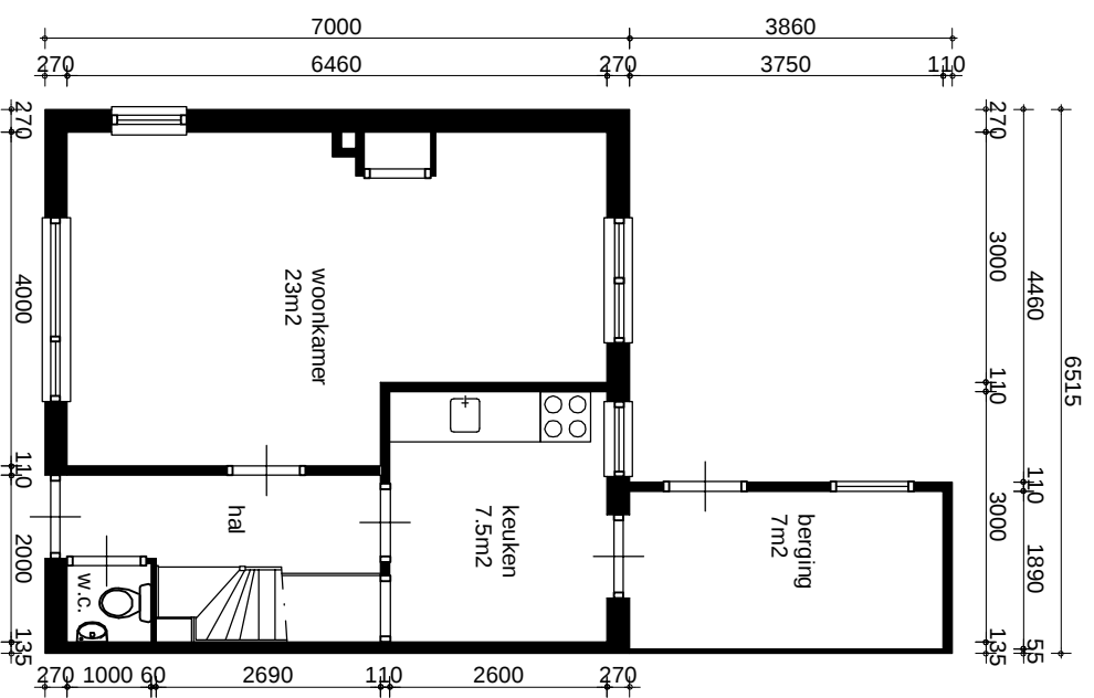
Begane grond
