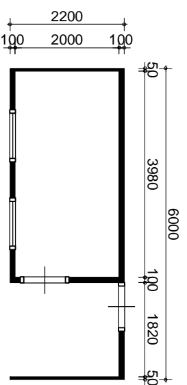
Platte grond
