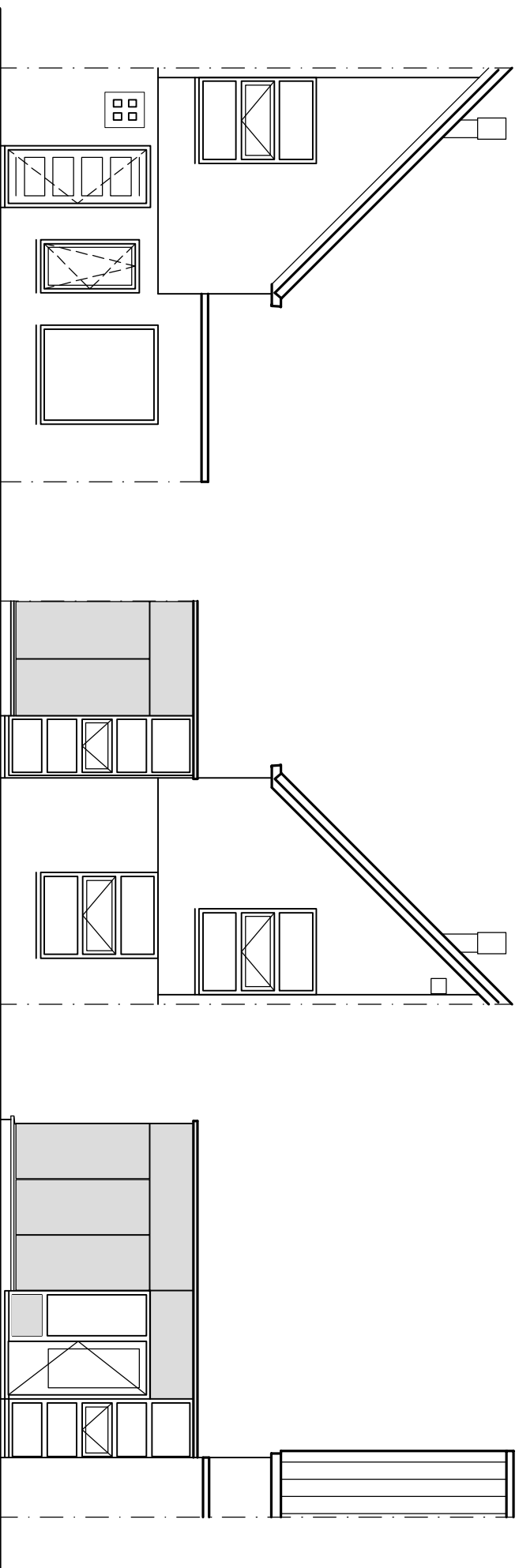
Voorgevel
