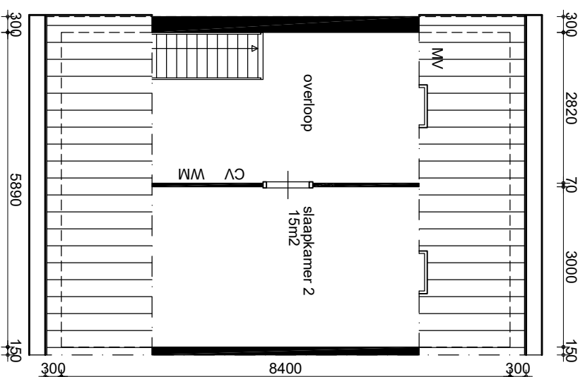
Verdieping
