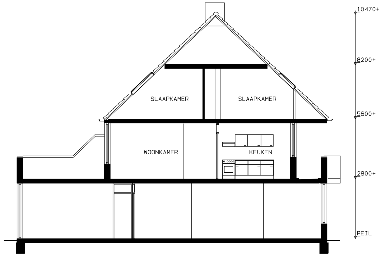
DOORSNEDE
