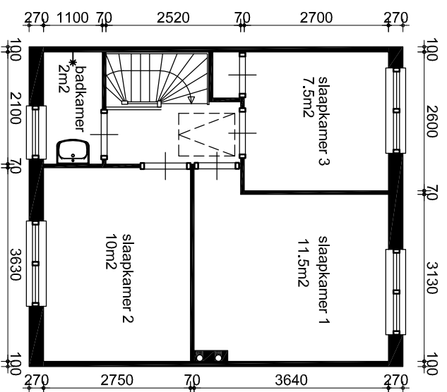
Verdieping
