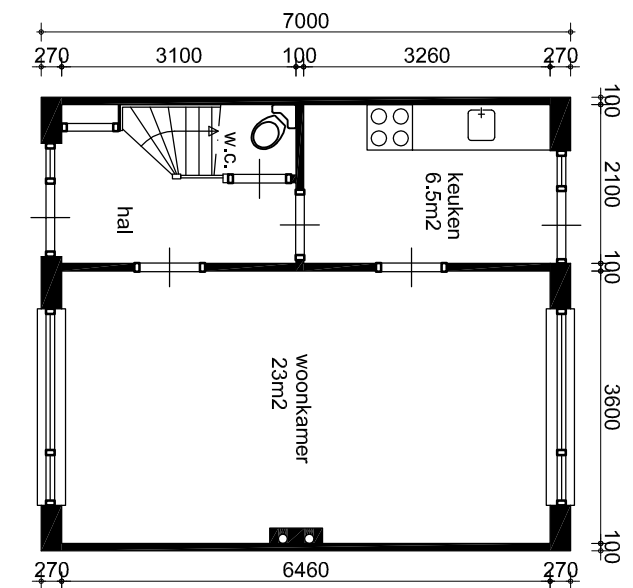
Begane grond
