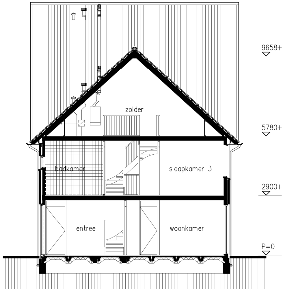
Doorsnede
