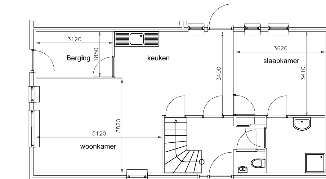
beganegrond
