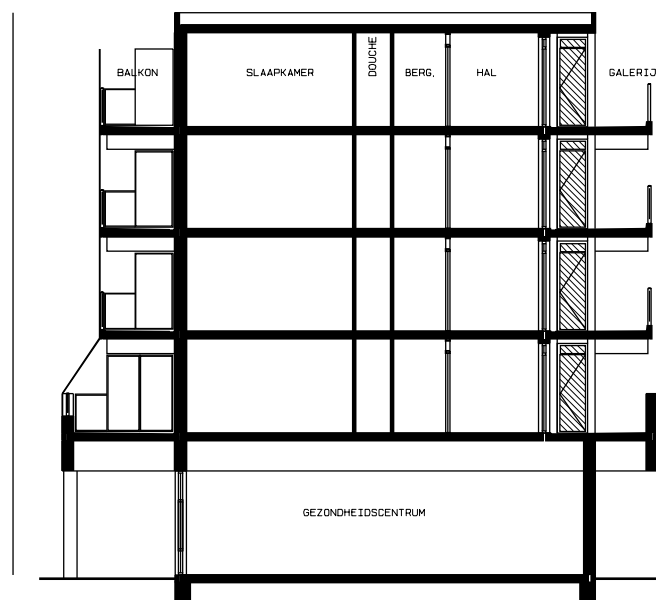
DOORSNEDE
