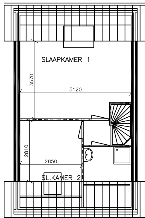
1e Verdieping
