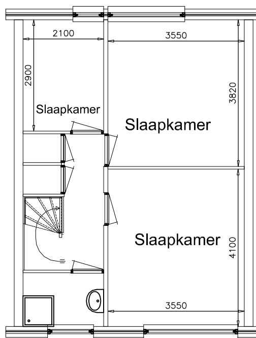
1e verdieping
