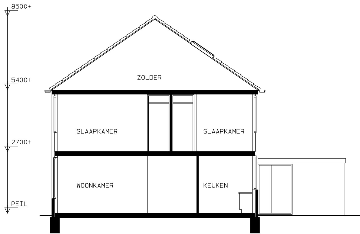
DOORSNEDE
