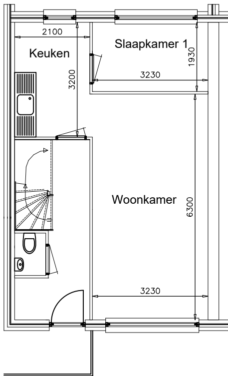
1e verdieping
