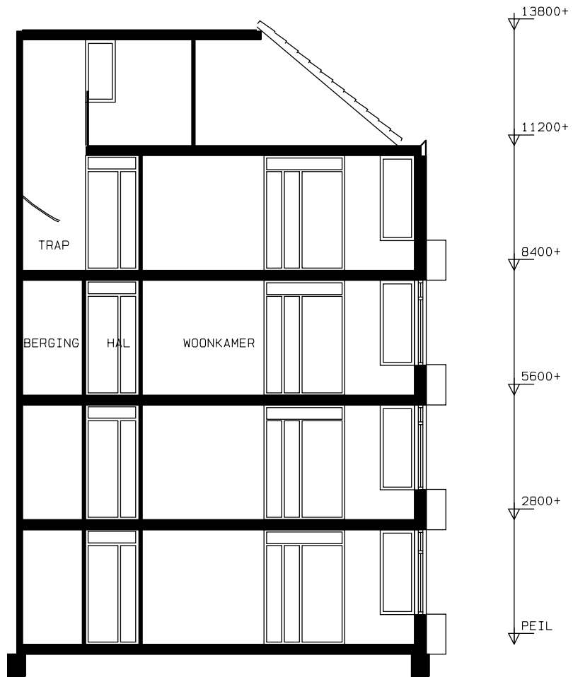
DOORSNEDE
