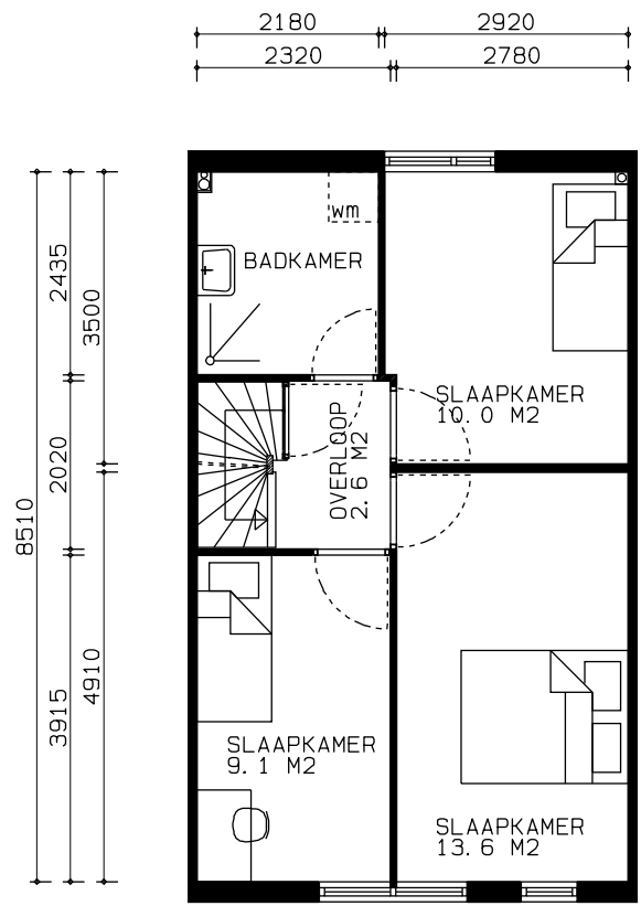
1e VERDIEPING
