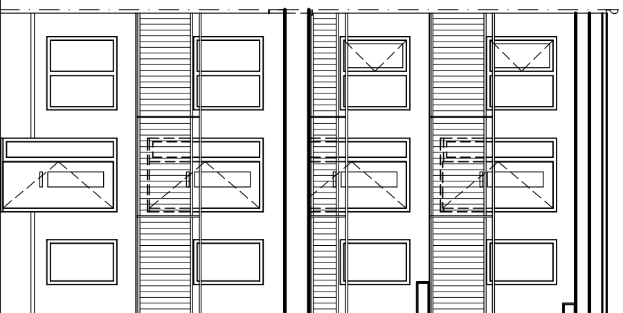
Binnengevel
