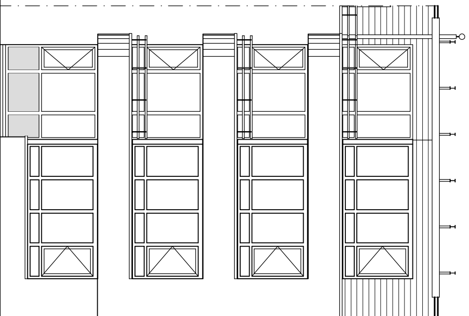
Voorgevel
