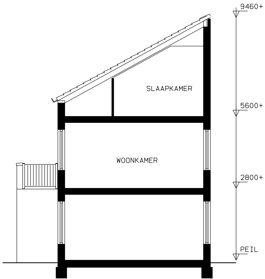
DOORSNEDE
