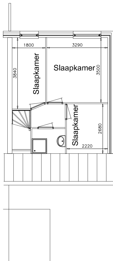
1e verdieping
