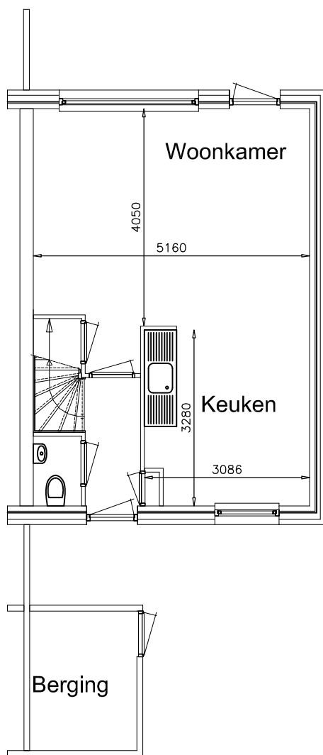
begane grond
