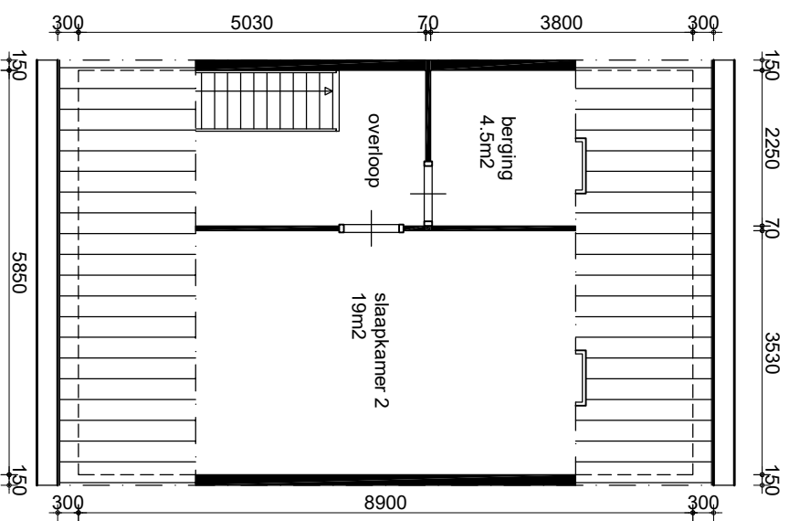
Verdieping
