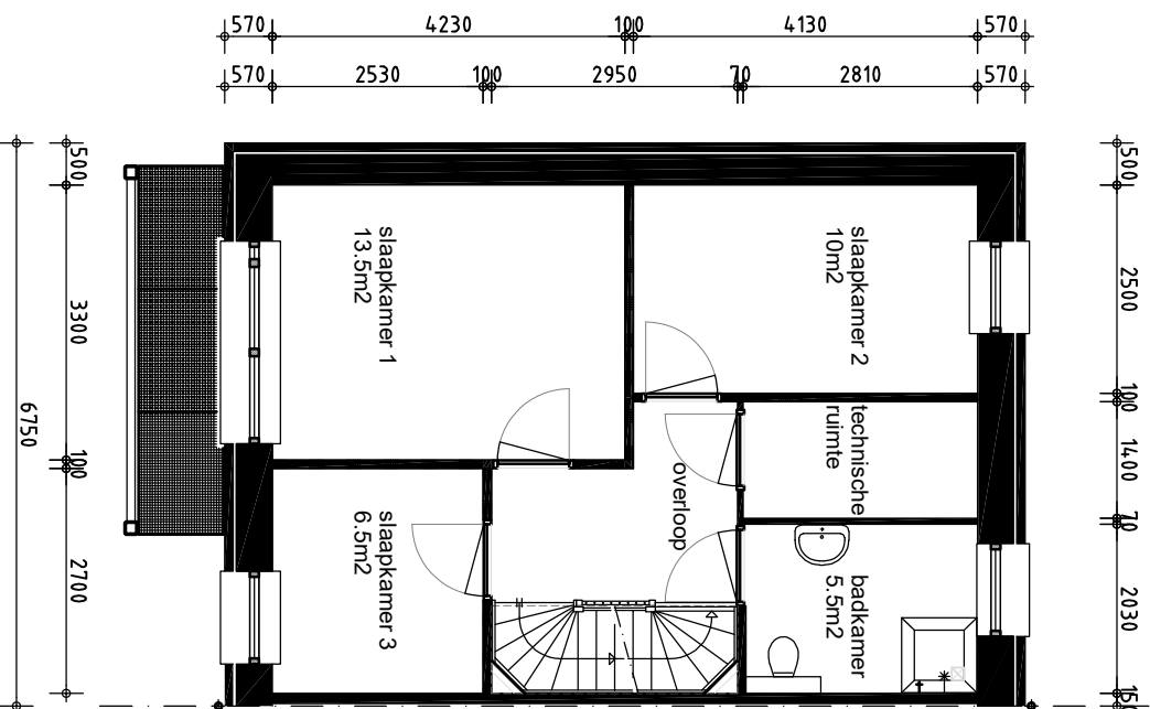
Verdieping
