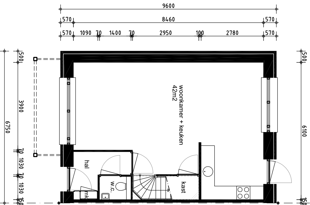
Begane grond
