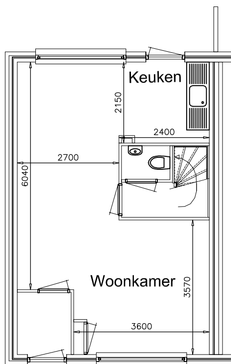
Begane grond
