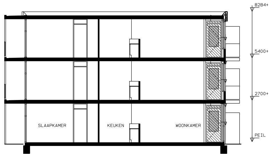
DOORSNEDE
