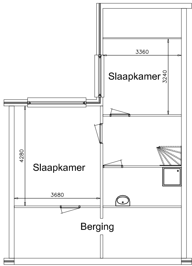
1e verdieping
