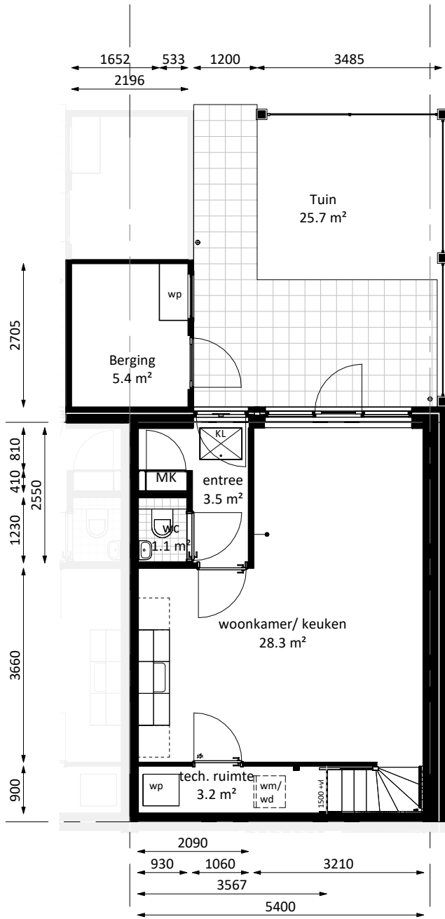
begane grond
