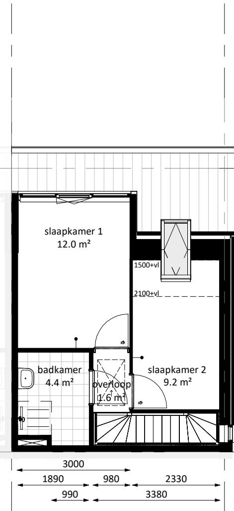
eerste verdieping
