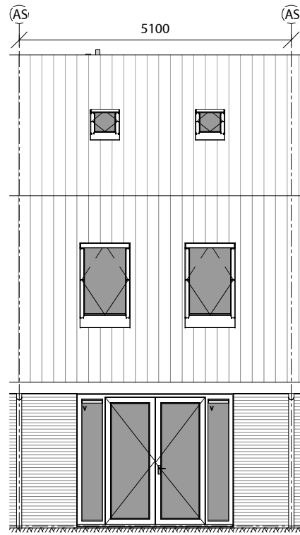
achtergevel
