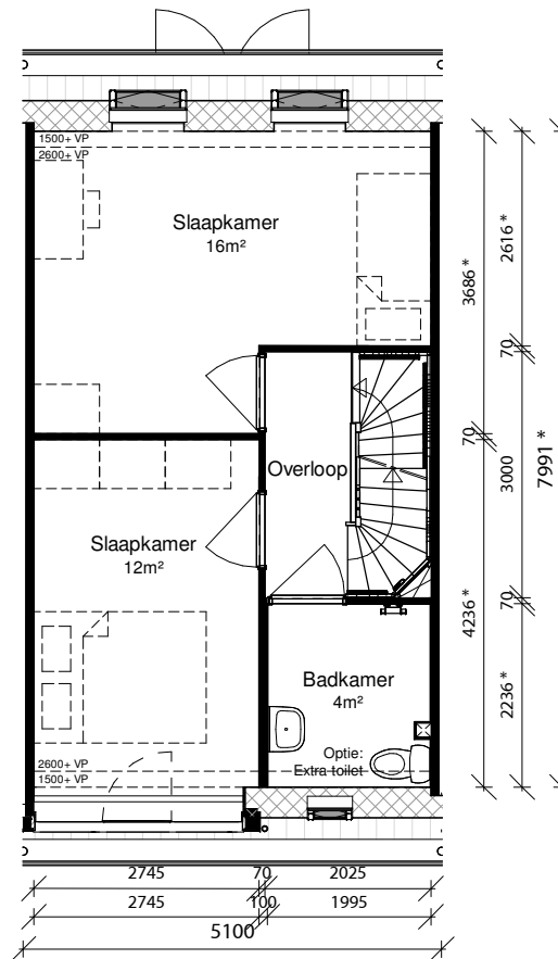
1e verdieping
