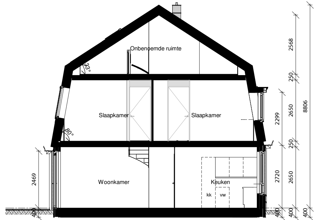
Doorsnede
