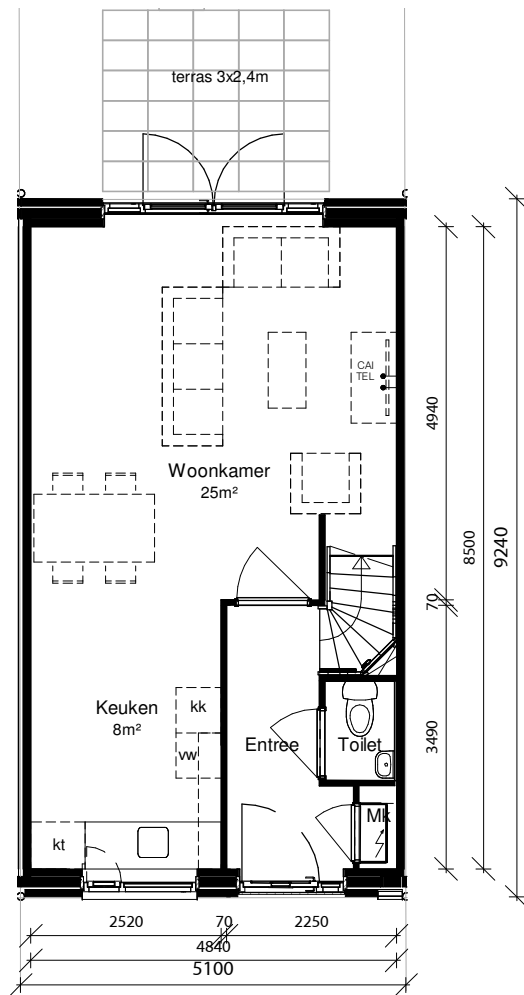
begane grond
