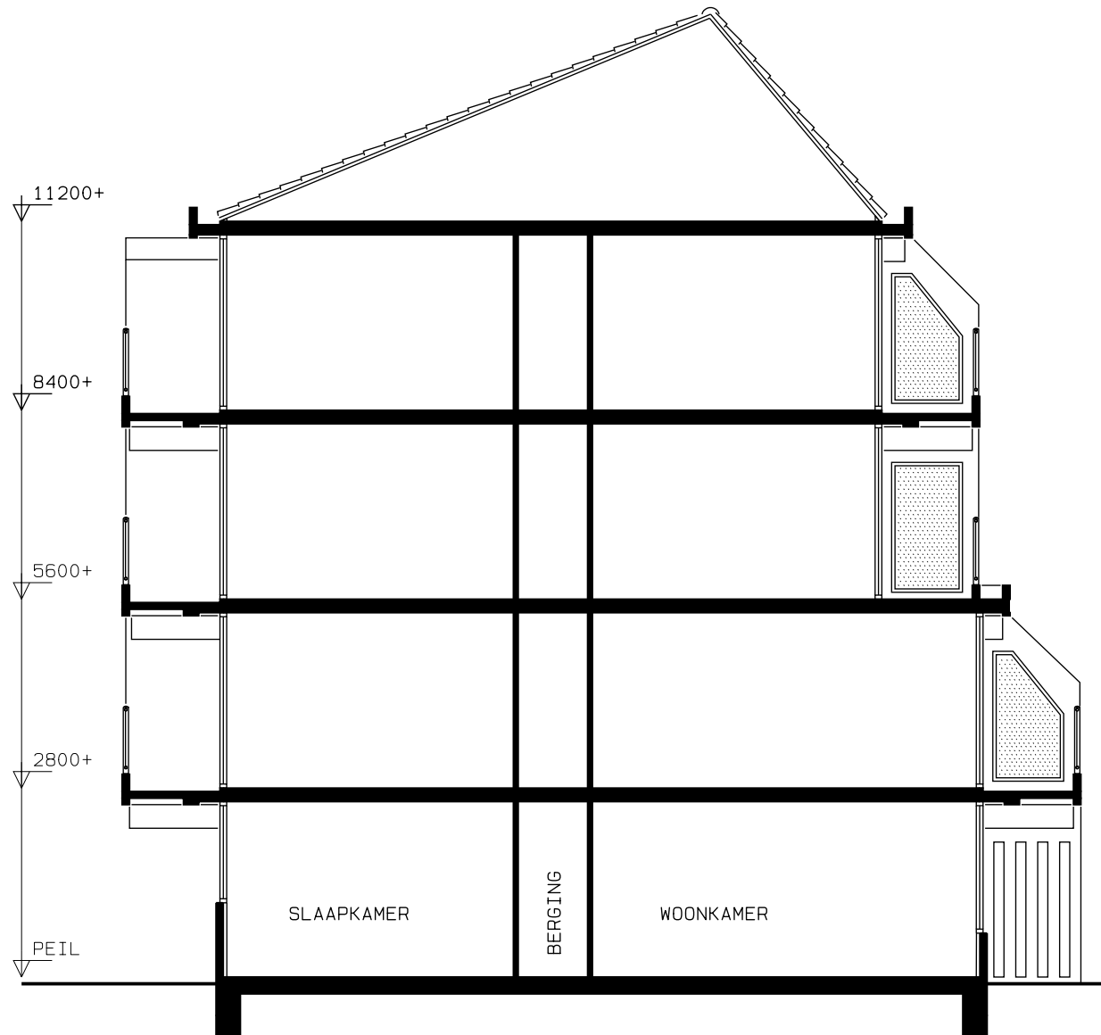
DOORSNEDE
