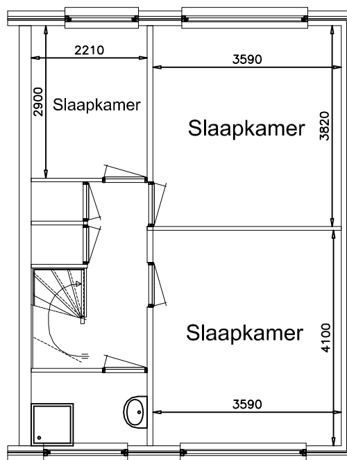
1e verdieping
