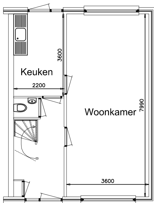
Begane grond
