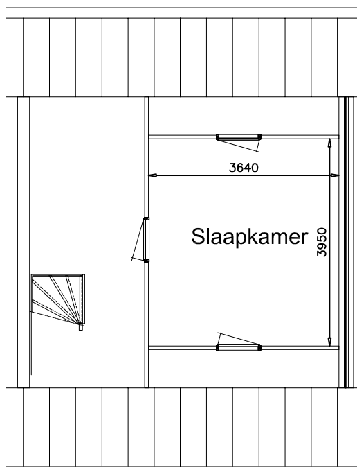
2e verdieping
