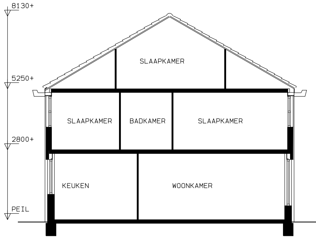
DOORSNEDE
